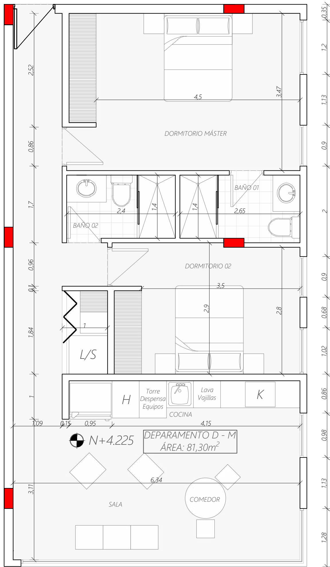
PLANTA DEPARTAMENTOS EN 1RA PA - 2DA PA - 3RA PA
